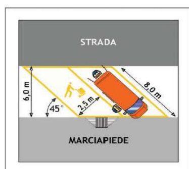
Figura 3 - Piazzola a 45°
